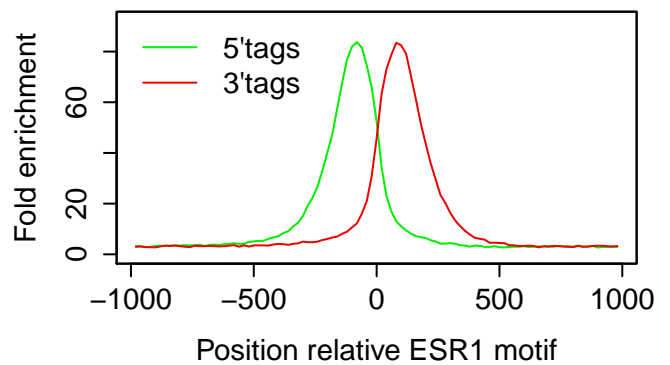
T47D|ESR1|Progesterone 3hr|rep3
