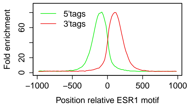
MCF7|ESR1|E2 3hr|rep3
