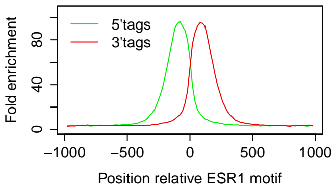
T47D|ESR1|Full_Media 3hr|rep1
