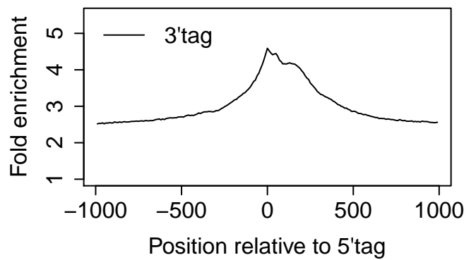
MCF7 | AR | |
